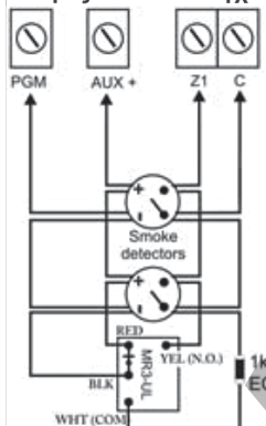
4-καλωδίων εγκατάσταση Κλέμες Πίνακα Ελέγχου
