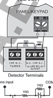
N.C. Επαφές, Με EOL, με Tamper & αναγνώριση σφάλματος καλωδίωσης (UL/ULC)
