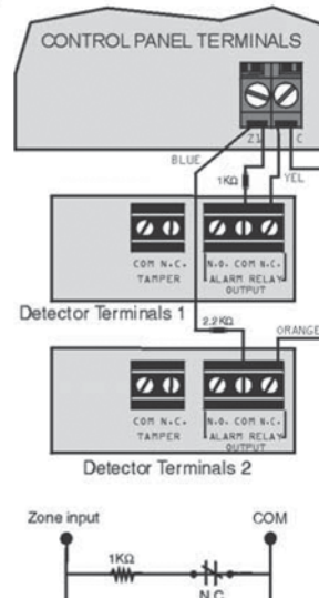
Παράλληλη Καλωδίωση
