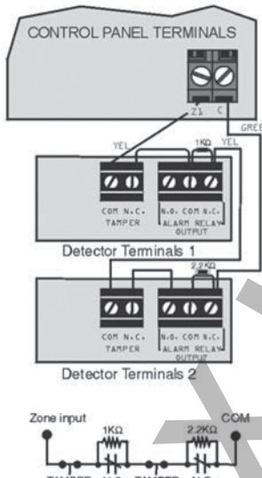
N.C. Επαφές, Χωρίς EOL, με αναγνώριση Tamper
