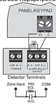
N.O. Επαφές, Με EOL UL/ULC Παραμετροποίηση
