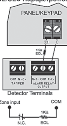
N.C. Επαφές, Με EOL UL/ULC Παραμετροποίηση
